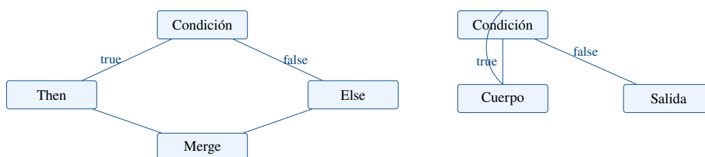
Figura 6.3: CFG generado para if-else (izquierda) y while (derecha).
